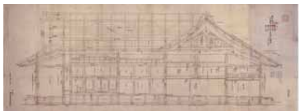
御本丸大広間南御入側より御上段後御入側二十分ノ一総建地割
